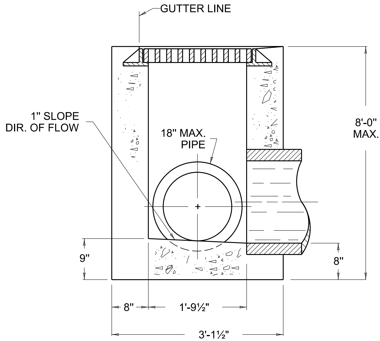
SECTION A-A
